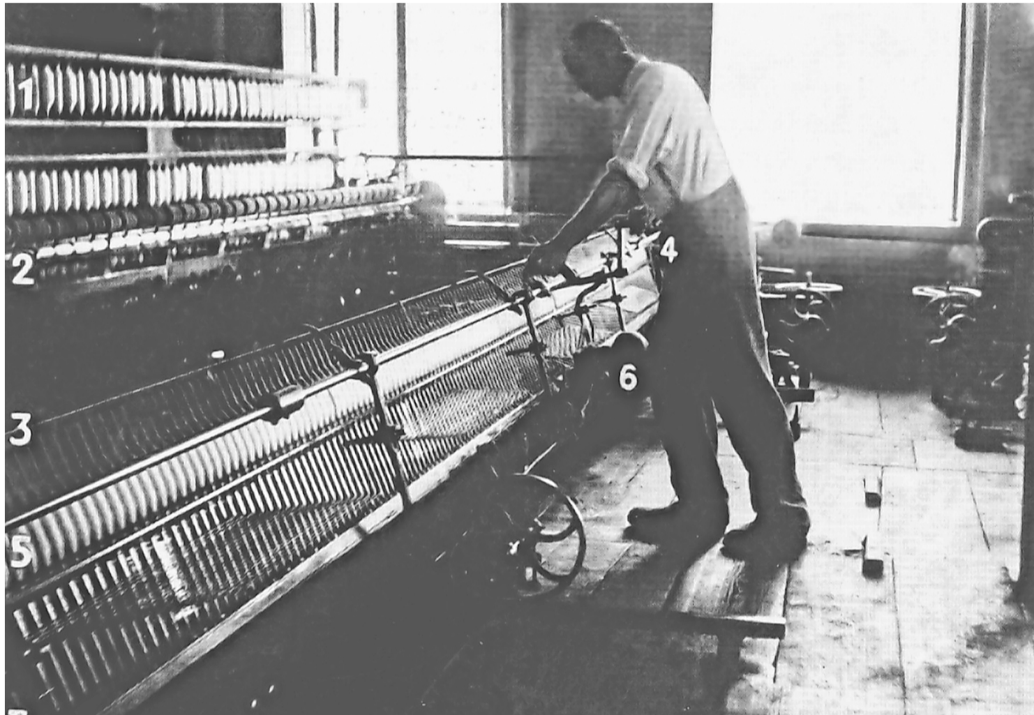
Ein Fabrikarbeiter (um 1900) an einem sogenannten Halbselfaktor, mit welchem schon vor rund 180 Jahren im grossen Stil feinste Garne hergestellt werden konnten. Archivbild: Kläui/Hinwil aus dem Buch «Spinnerkönig Heinrich Kunz»
