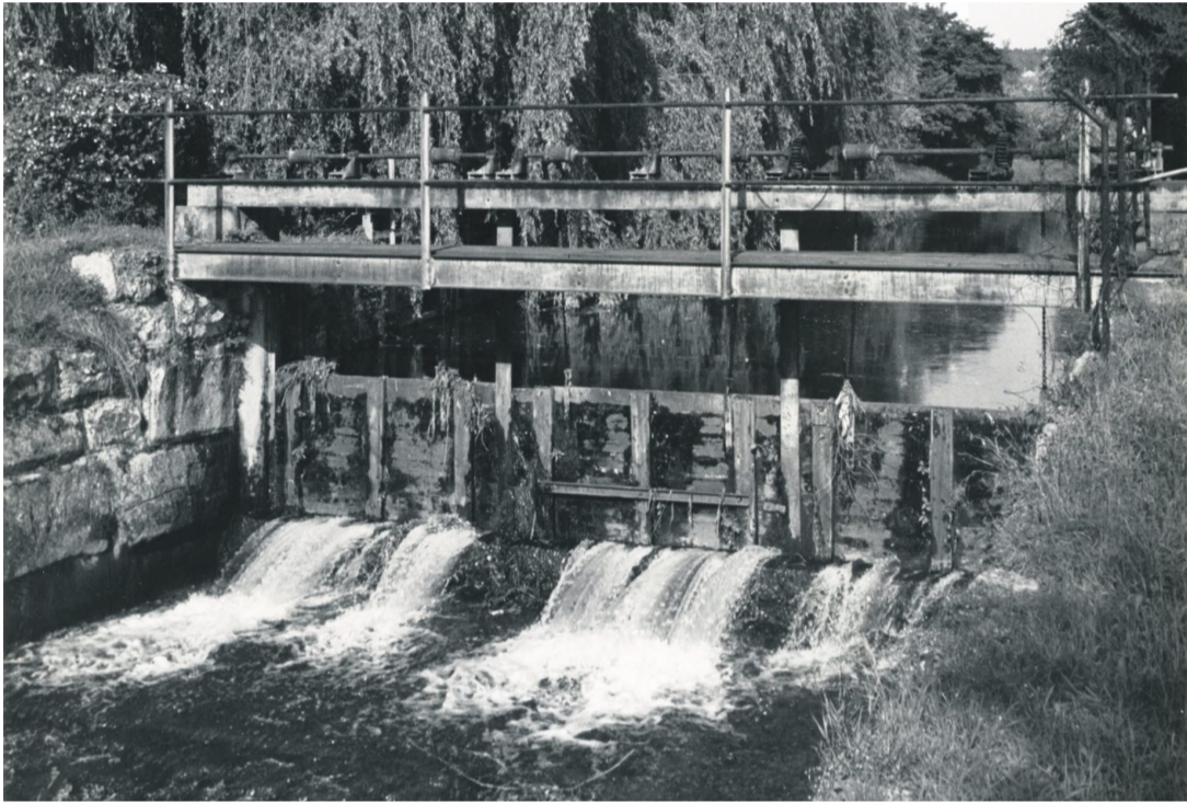
Wasserkraft trieb die Spinnstühle an. Stauwehr beim heutigen Stadtpark von Uster.
